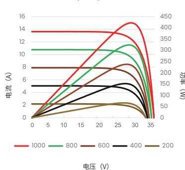
电流 - 电压 & 功率 - 电压曲线图 (435W)
