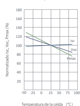
Dependencia de temperatura de I sc , V oc , P max
