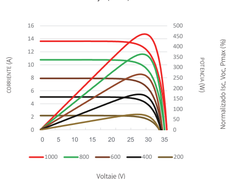
Curvas de corriente-voltaje y potencia-voltaje (470W)
