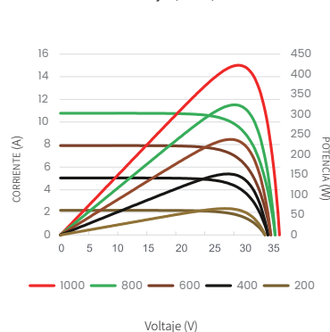
Curvas de corriente-voltaje y potencia-voltaje (435W)
