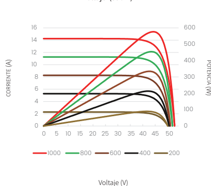
Curvas de corriente-voltaje y potencia-voltaje (590W)
