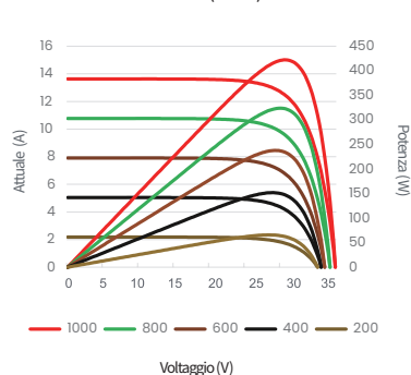
Curve corrente-tensione e potenza-tensione (435W)
