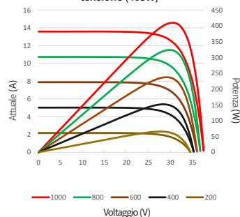
Curve corrente-tensione e potenza-tensione (405W)
