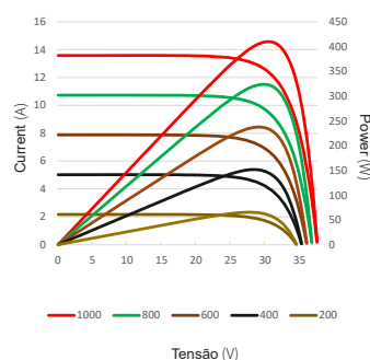
Curvas de corrente-tensão e potência-tensão (410W)
