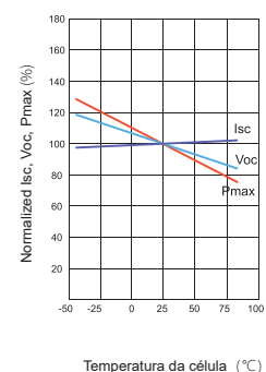
Dependência de temperatura de I_{sc} , V_{oc} , P_{max}
